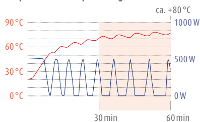
Temperaturverlauf / Leistungsaufnahme
